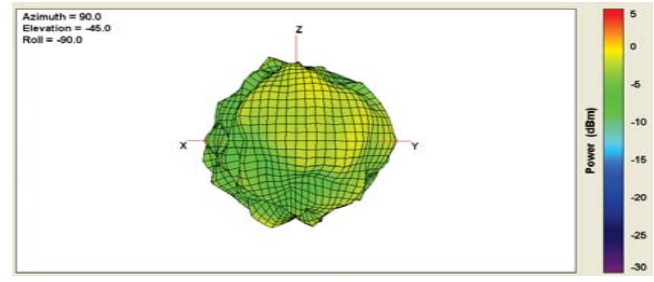
3D 5500MHz
