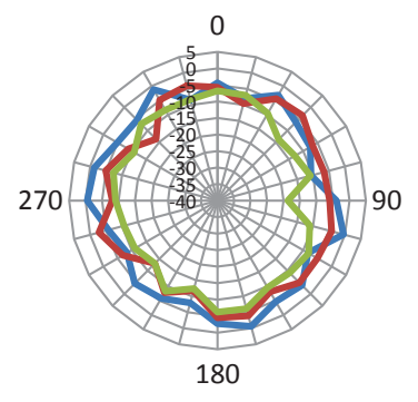
2D XOZ
