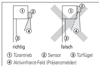
Seitenansicht
