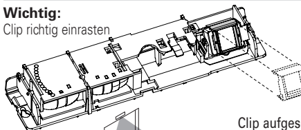
Clip aufgesetzt
