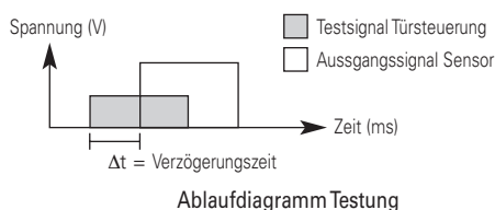
Ablaufdiagramm Testung
