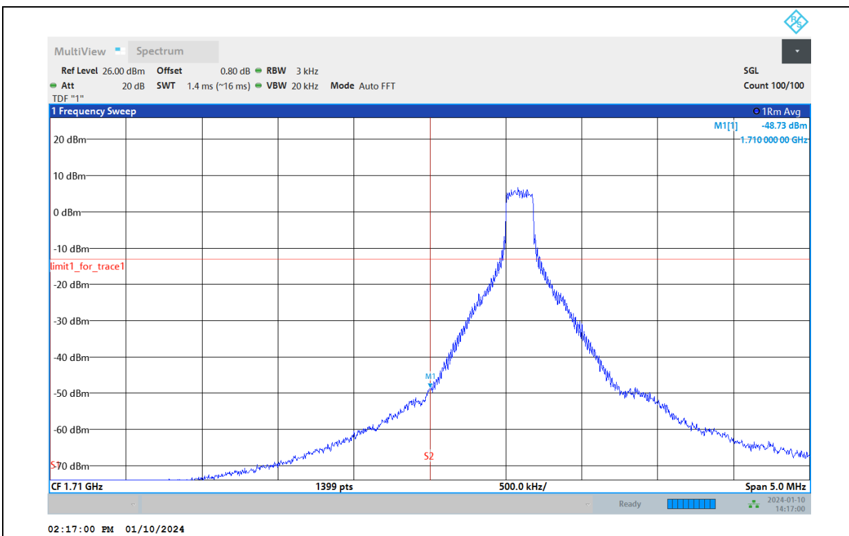
Band66-10MHz-QPSK-132022-50RB#0
