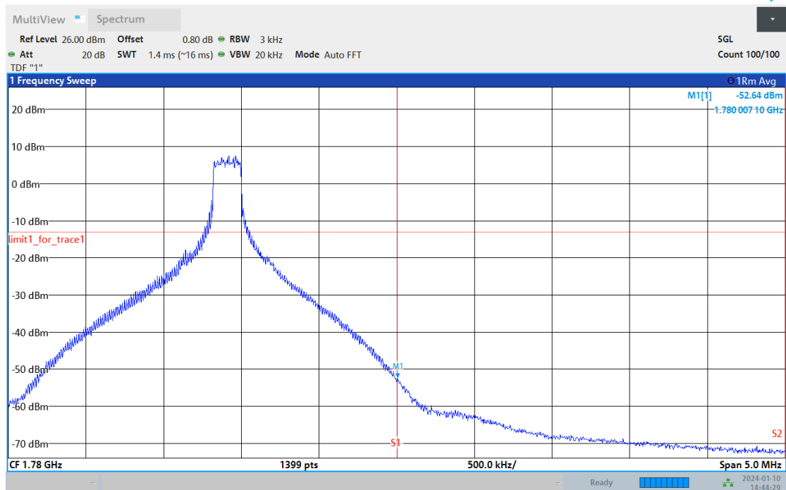
Band66-20MHz-QPSK-132572-100RB#0
