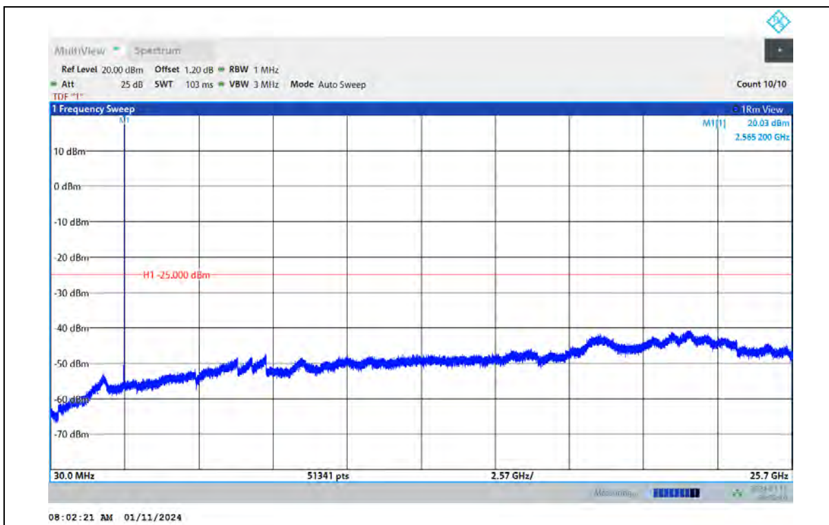
Band7-10MHz-QPSK-20800-1RB#0-Range:30~25700MHz
