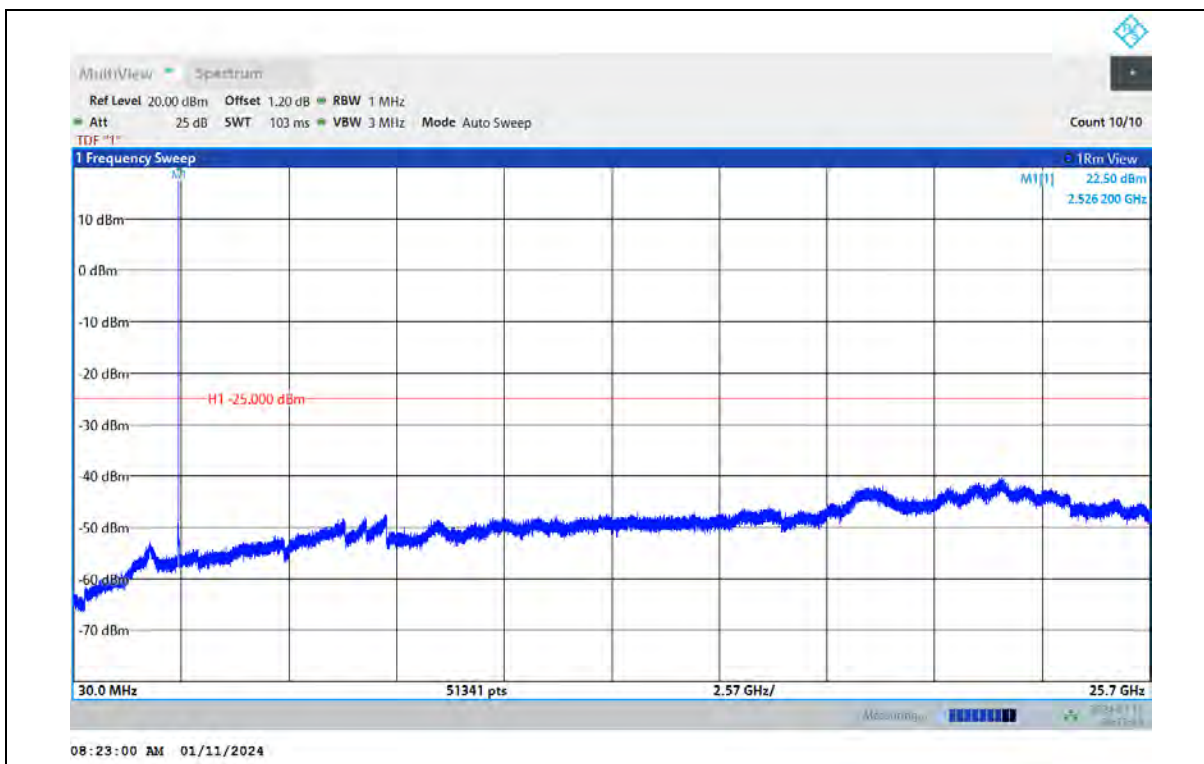
Band7-20MHz-QPSK-21350-1RB#0-Range:30~25700MHz
