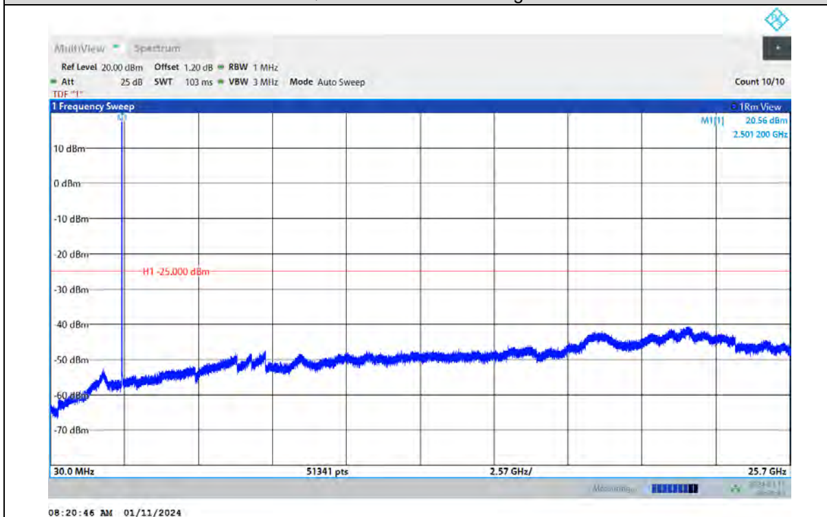
Band7-20MHz-QPSK-21100-1RB#0-Range:30~25700MHz
