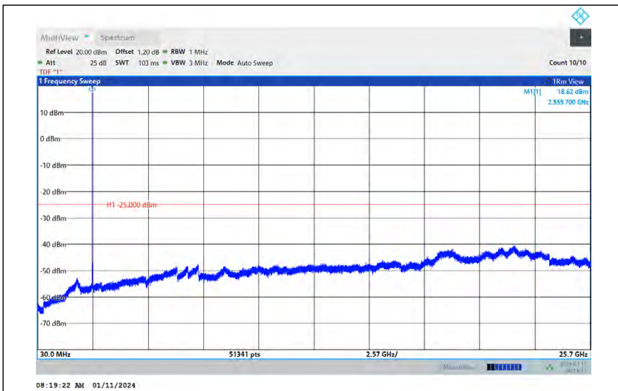
Band7-20MHz-QPSK-20850-1RB#0-Range:30~25700MHz
