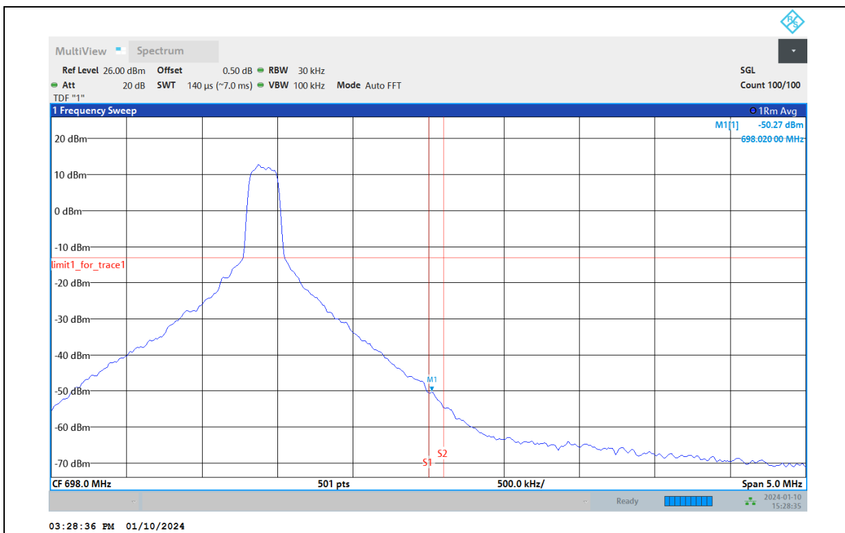
Band71-20MHz-QPSK-133372-100RB#0
