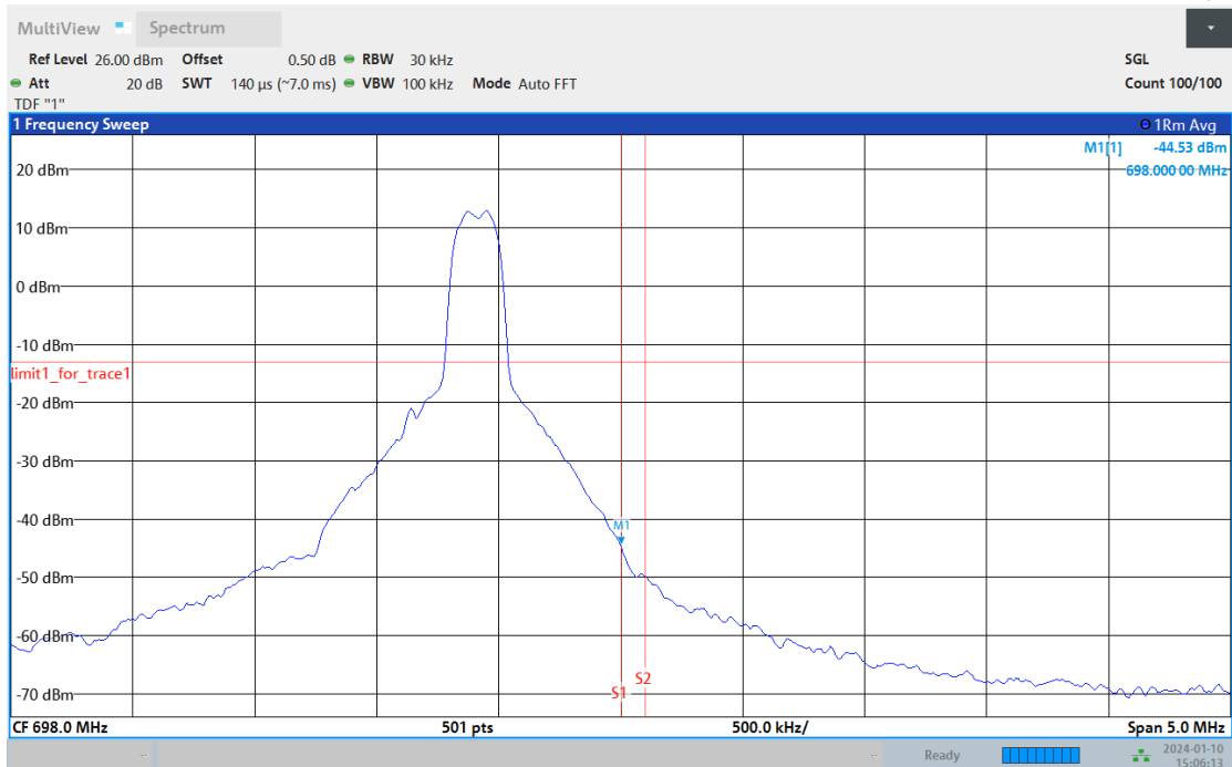
Band71-10MHz-QPSK-133422-50RB#0
