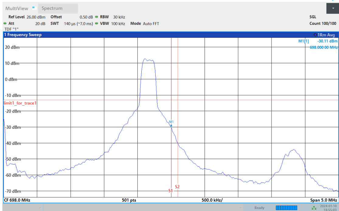
Band71-5MHz-QPSK-133447-25RB#0
