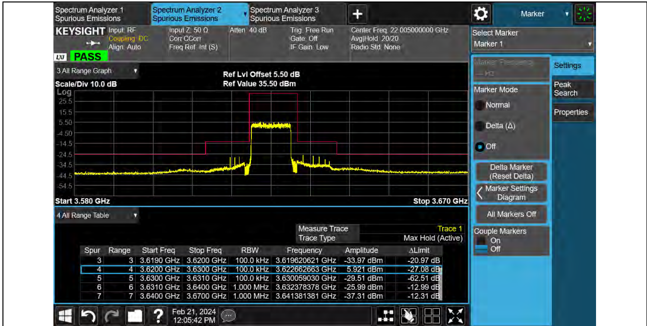
Band48-10MHz-QPSK-56690-1RB#0
