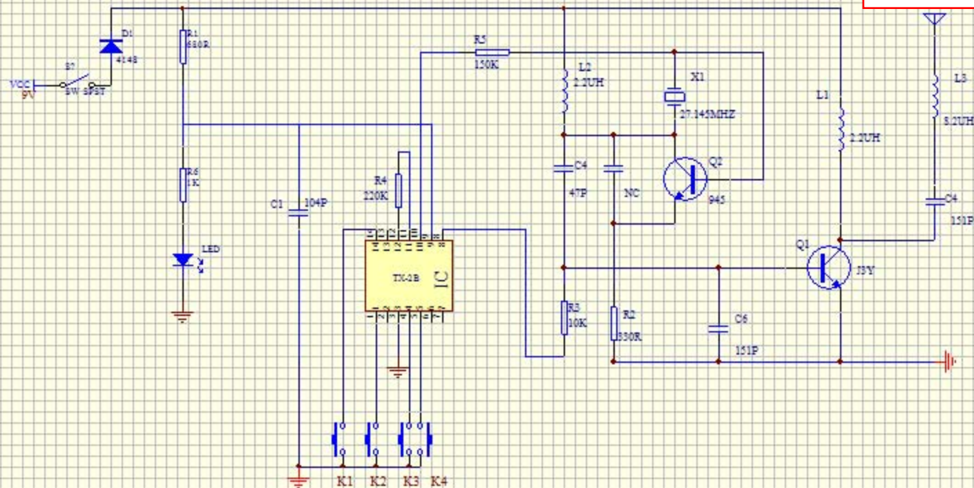
JR-452TX 27M发射原理图
