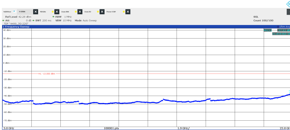
Diagram 3.1c, WCDMA TM1, LTE: E-TM1.1, Bim W+L , 3 GHz – 22 GHz, Port A:
