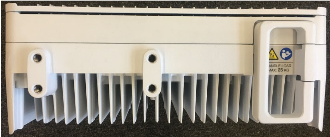
Top side
