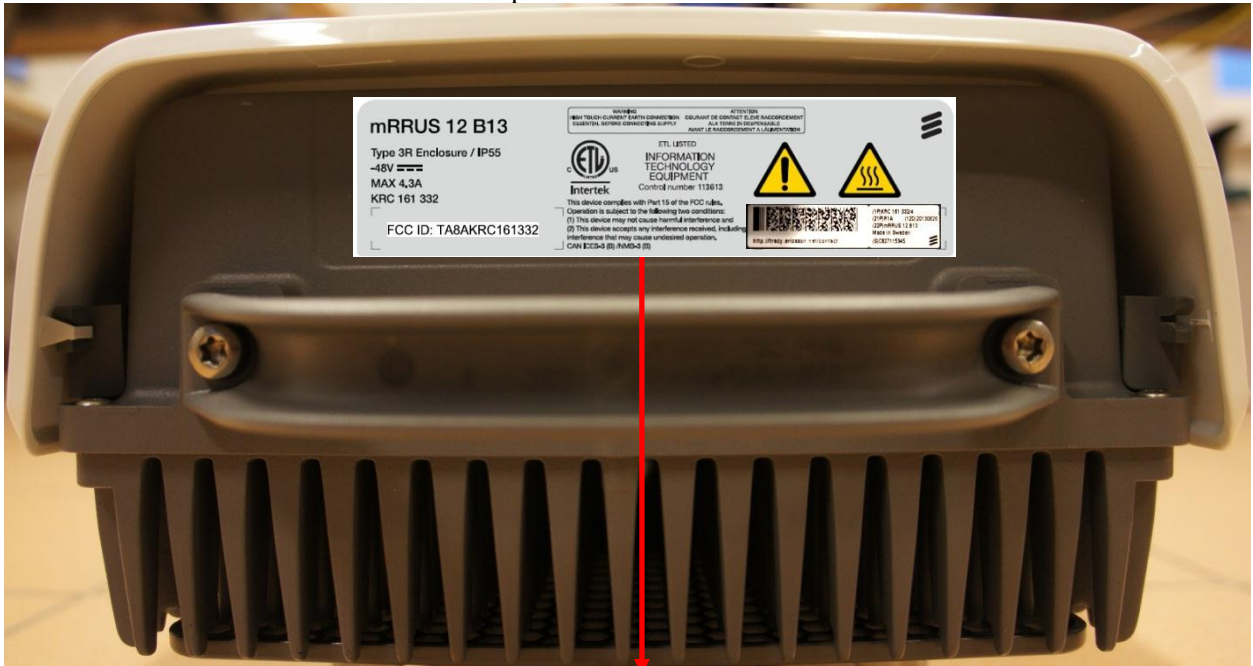
Top side KRC 161 332/4
