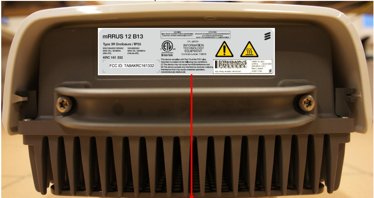
Top side KRC 161 332/3
