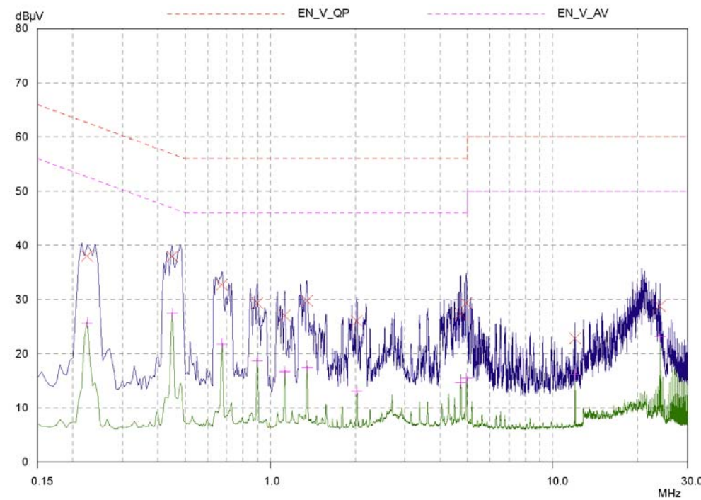
Neutral – PE
