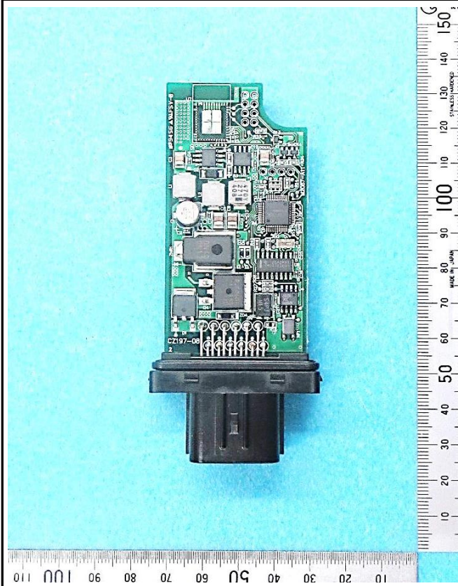
アンテナ内部 Inside the antenna
