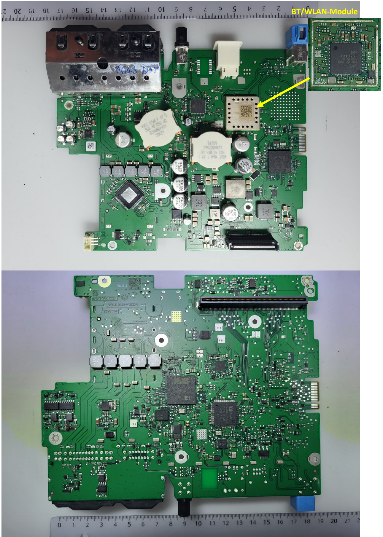
PCBA 4010 MAIN BB D15
