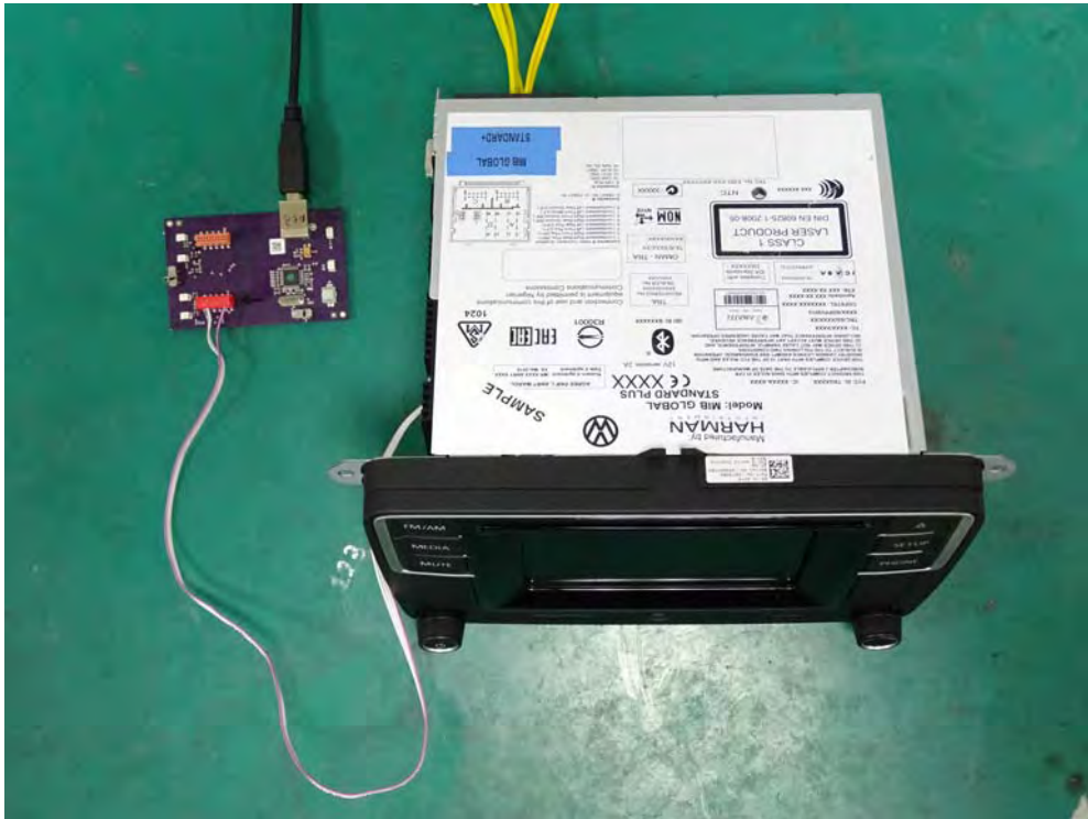
EUT & Test Fixture
