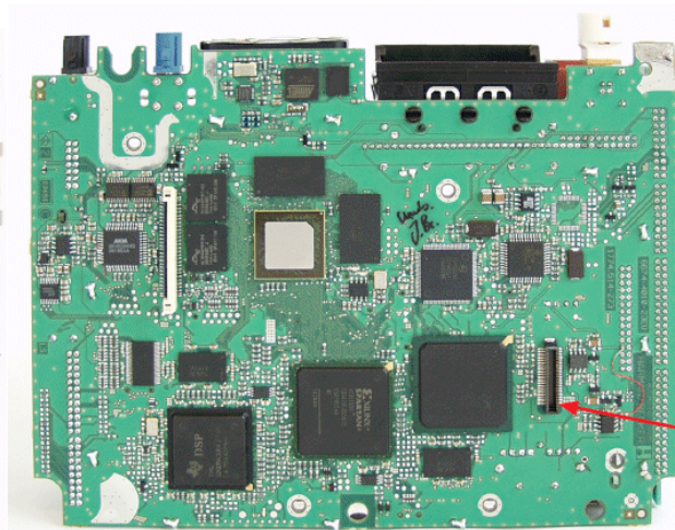
Mainboard 7675-4010-ls
