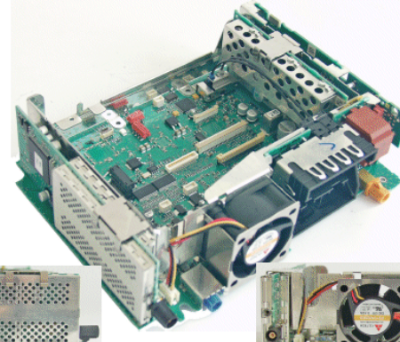
Konnektorboard 4040-bs
