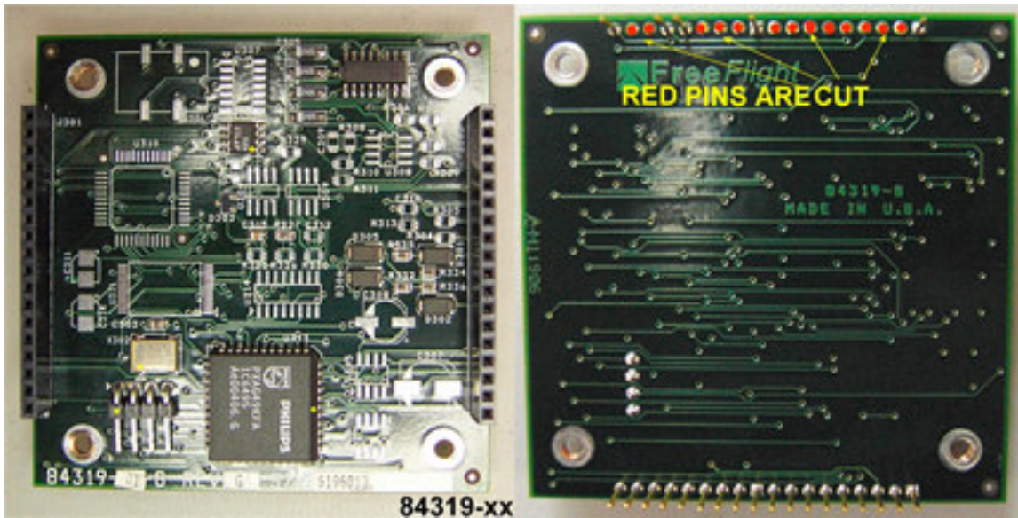
Fig 5 - 84319
