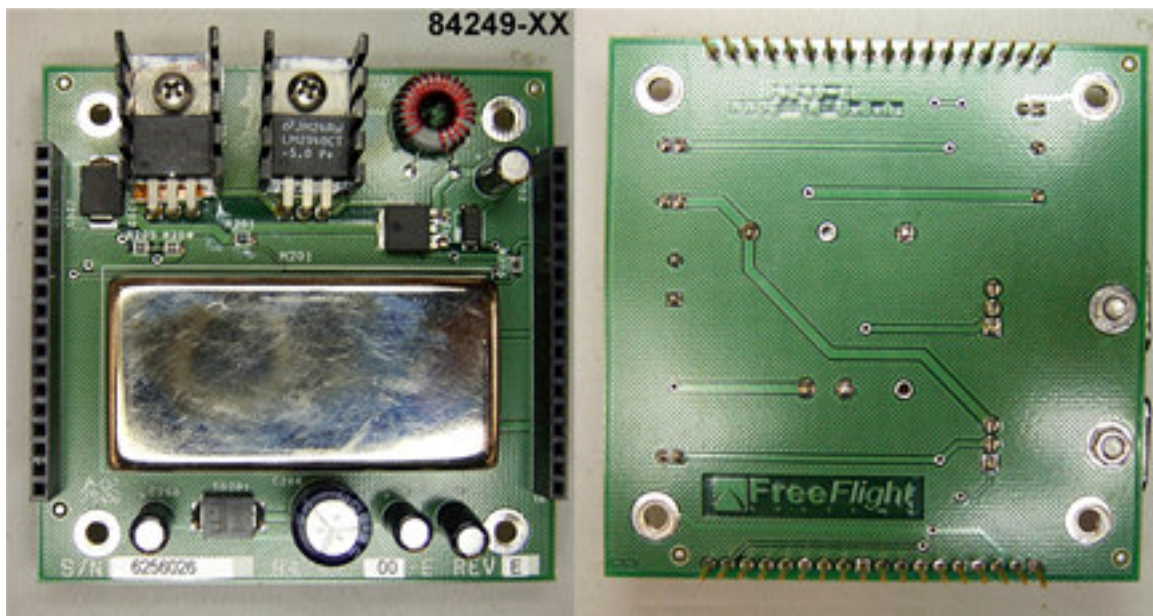
Fig 4 - 84249
