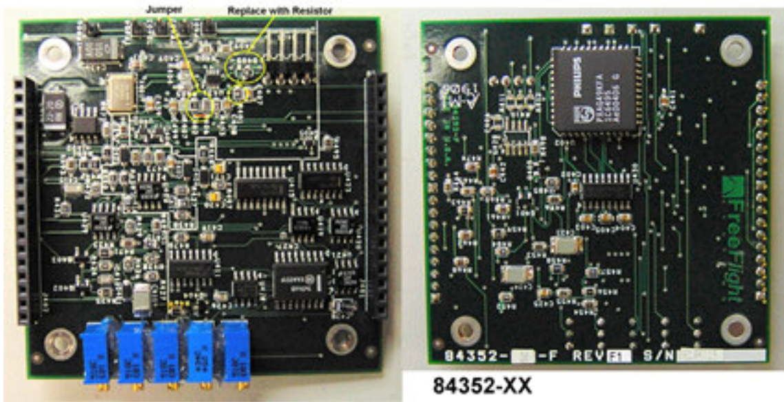
Fig 6 - 84352
