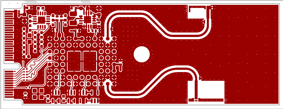
Layer 1 (Top)
