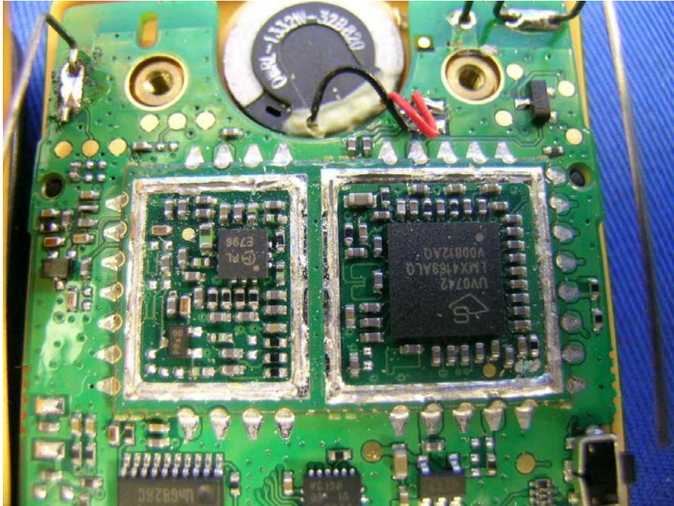
Handset 1.9G RF module
