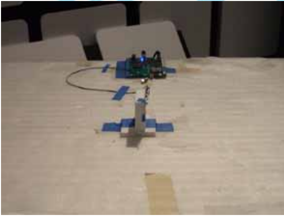
EUT Setup: WDAN-DQM3001-DF
