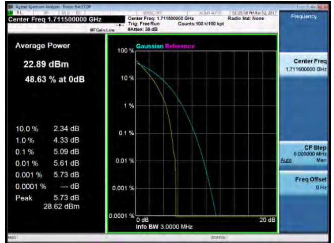
LTE_Band4 3MHz_16-QAM 15 0_LowCH19965-1711.5
