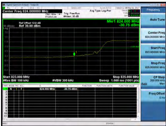
Band Edge_Band5_10MHz_QPSK_50_0_LowCH20450-829
