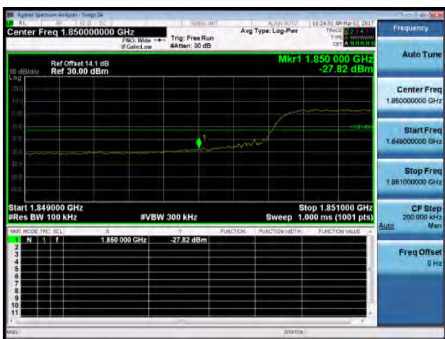
Band Edge_Band2_10MHz_QPSK_50_0_LowCH18650-1855
