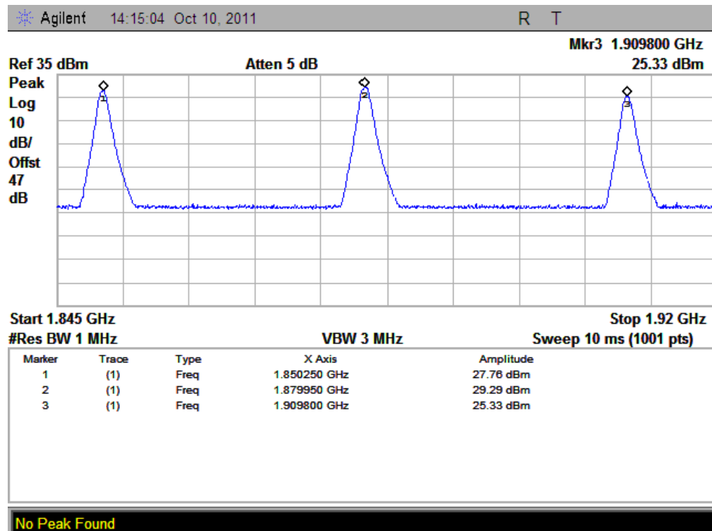
(Plot J: GPRS 1900MHz Channel = 512, 661, 810)
