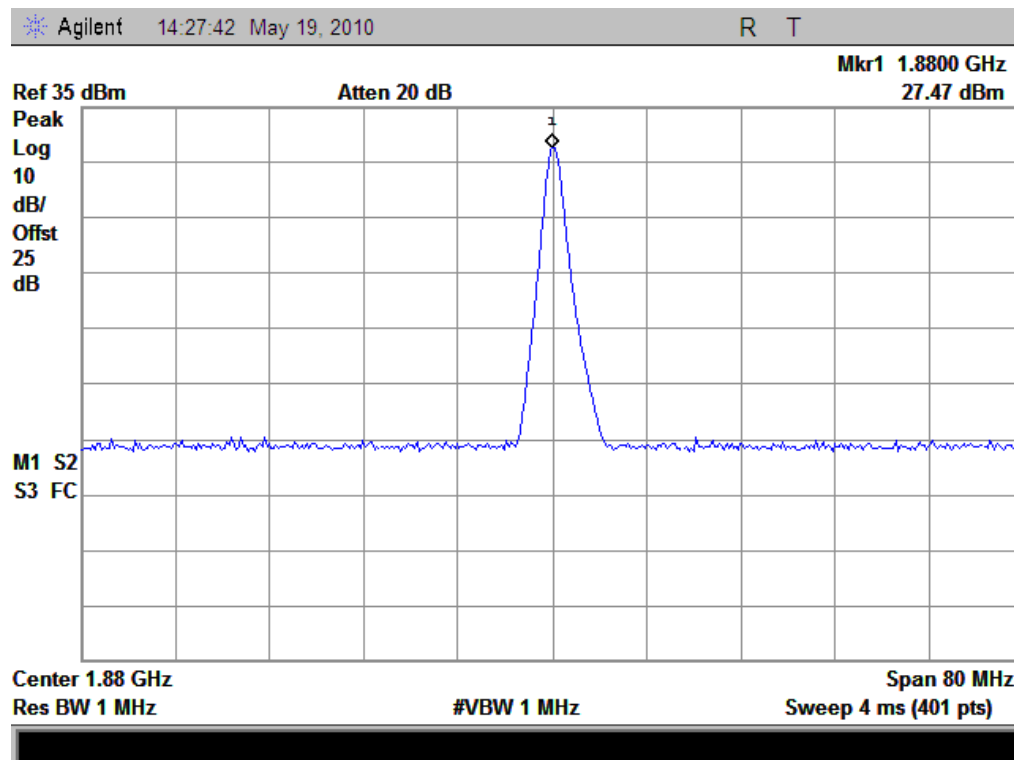
(Plot G: GPRS-2TX 1900MHz Channel = 661)
