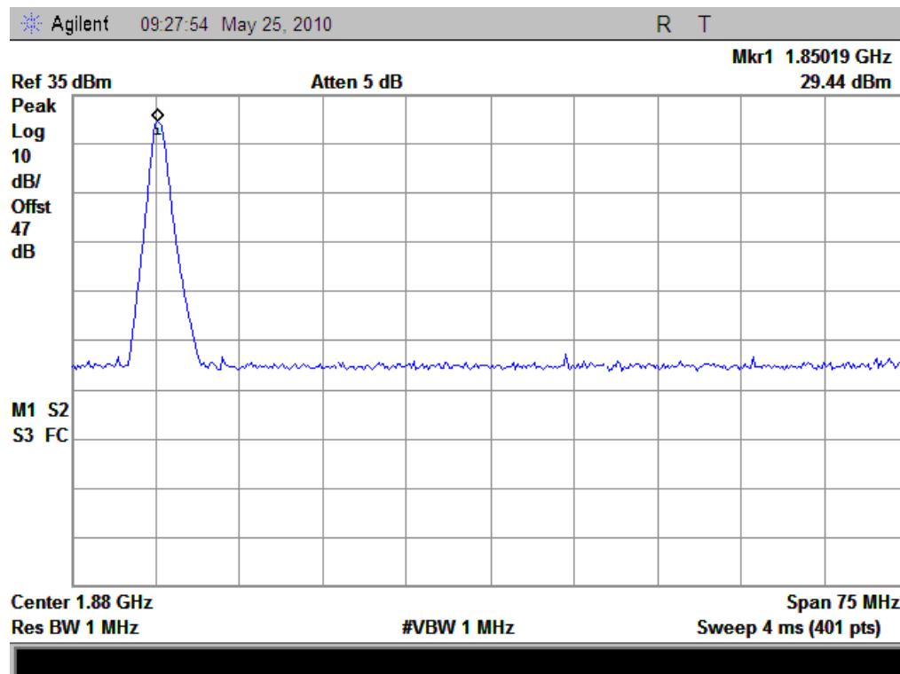
(Plot J: GPRS-2TX 1900MHz Channel = 512)
