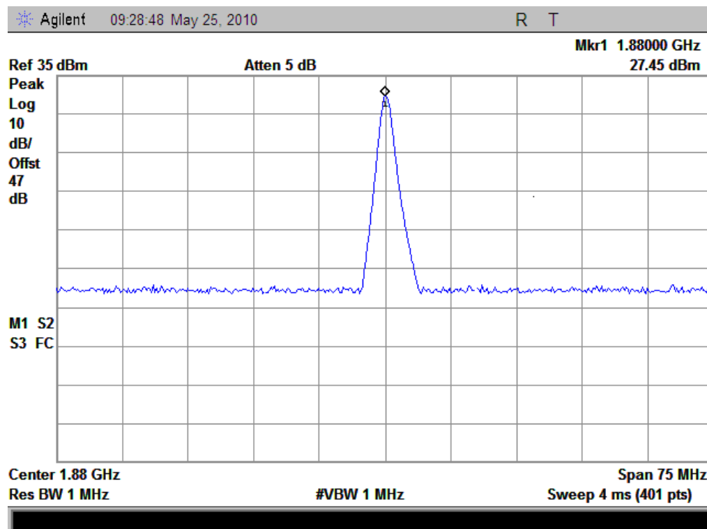
(Plot K: GPRS-2TX 1900MHz Channel = 661)
