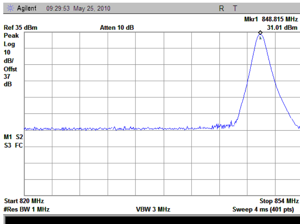
(Plot I: GPRS-2TX 850MHz Channel = 251)
