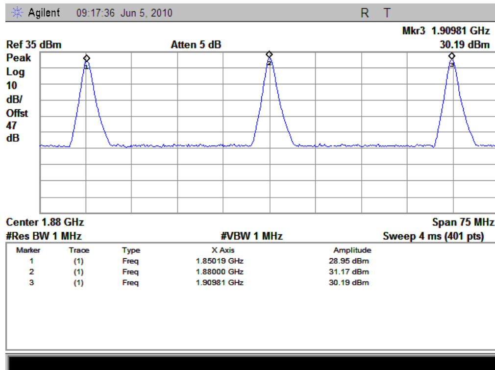
(Plot A: GSM 1900MHz Channel = 512, 661, 810)
