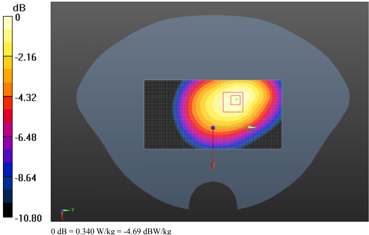
Fig. 7 850 MHz CH190
