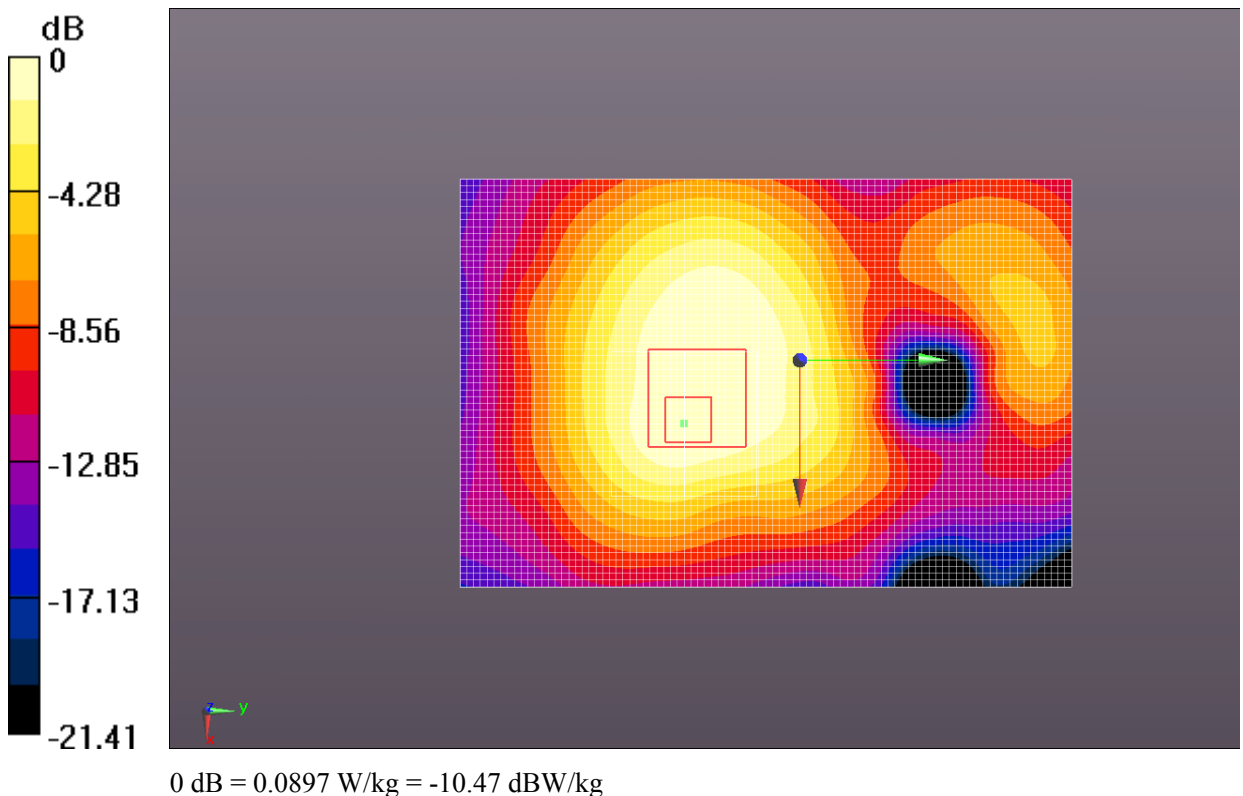
Fig. 35 2450 MHz CH1
