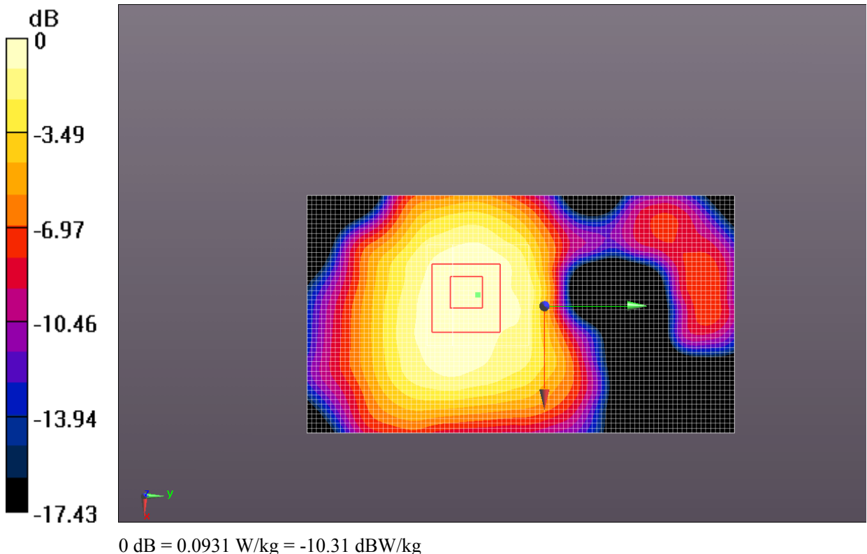
Fig. 37 2450 MHz CH6
