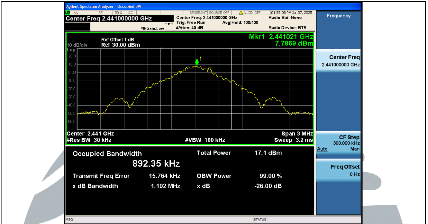
DH5-Ant1-2441
