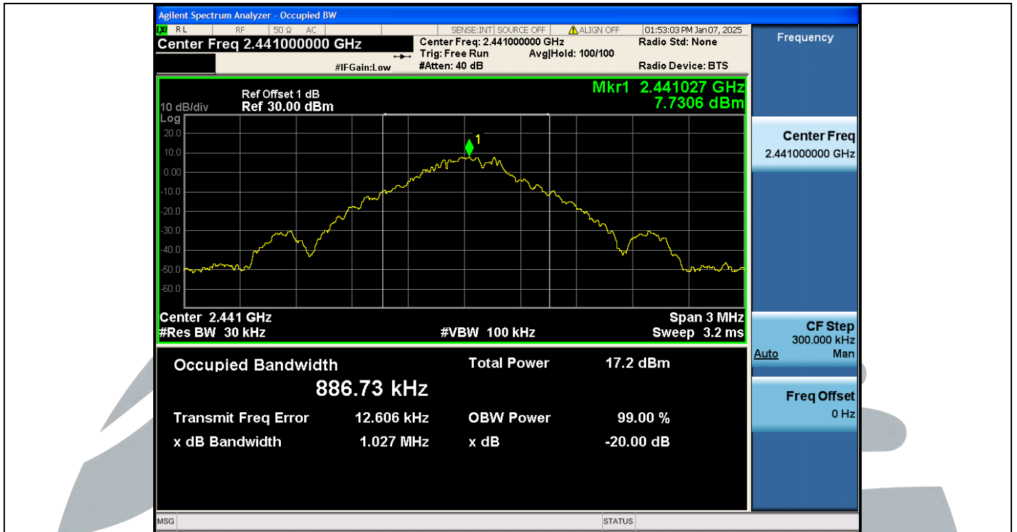
DH5-Ant1-2441
