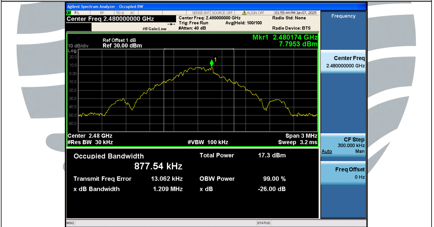
DH5-Ant1-2480
