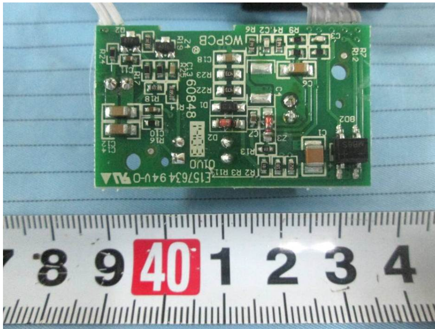
EUT – E15763494V-0 PCB Bottom View
