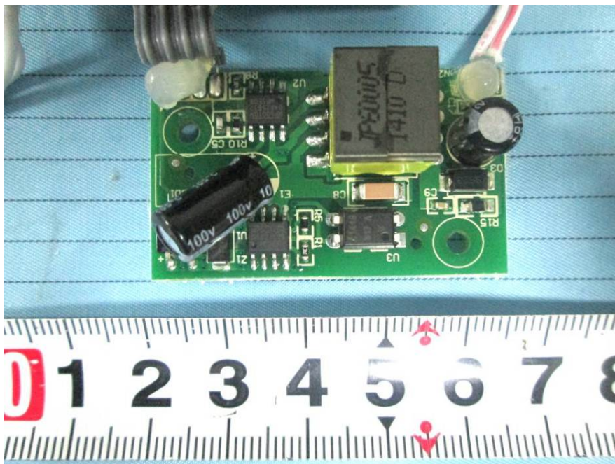
EUT – E15763494V-0 PCB Top View
