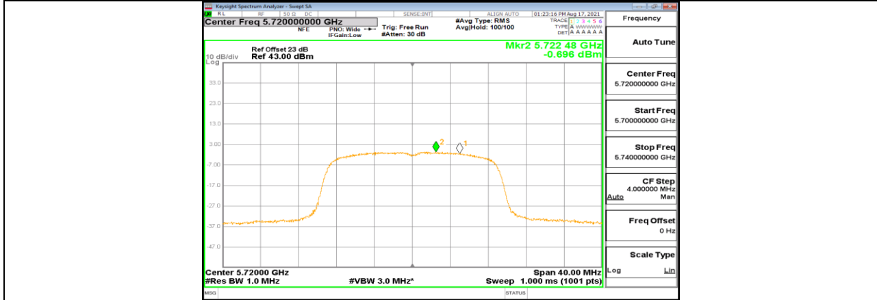
11N20MIMO_Ant2_5720_UNII-2C
