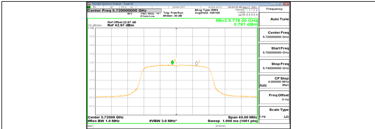
11A-CDD_Ant1_5720_UNII-2C
