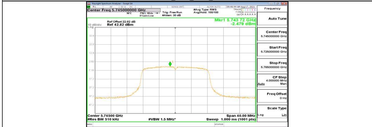
11A-CDD_Ant1_5745
