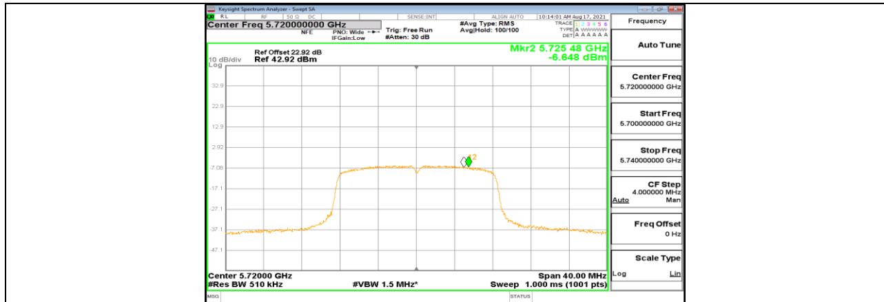
11A-CDD_Ant2_5720_UNII-3
