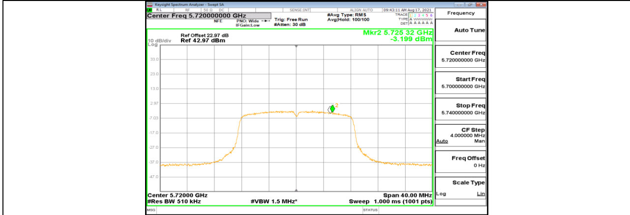
11A-CDD_Ant1_5720_UNII-3
