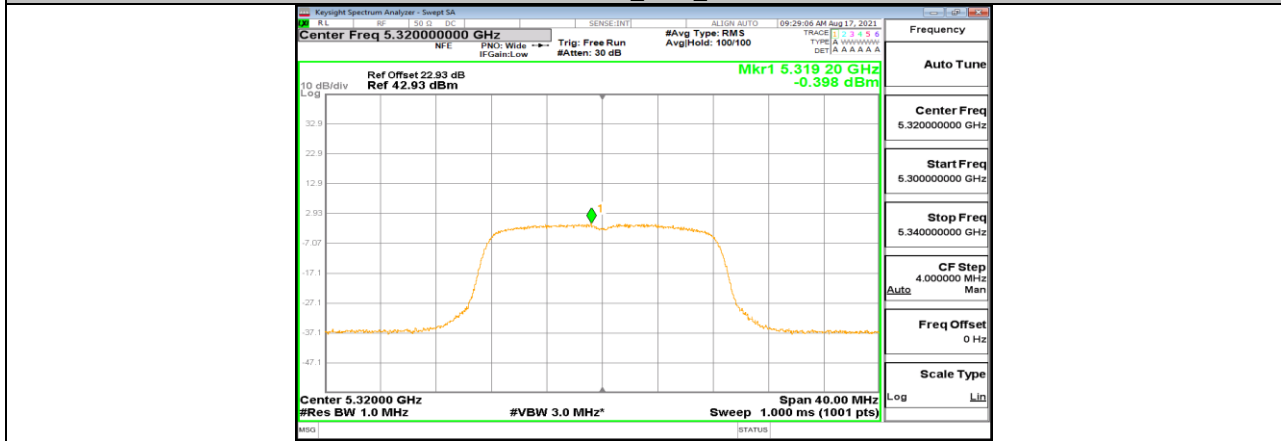
11A-CDD_Ant1_5320
