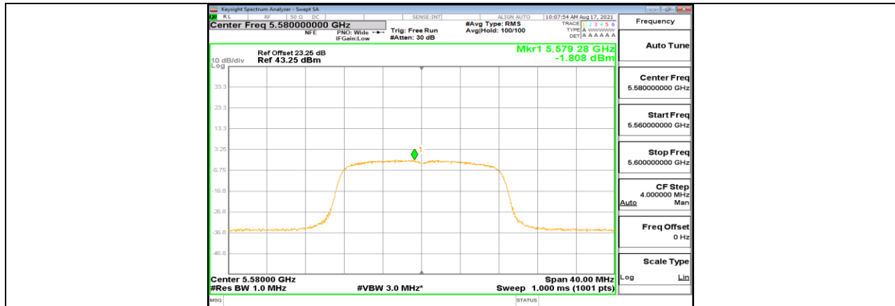
11A-CDD_Ant2_5580
