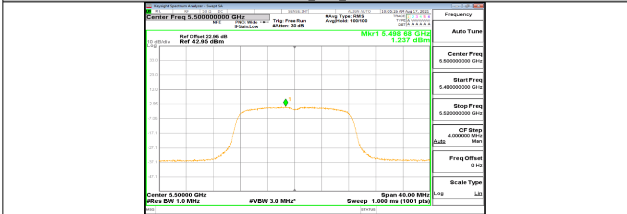
11A-CDD_Ant2_5500
