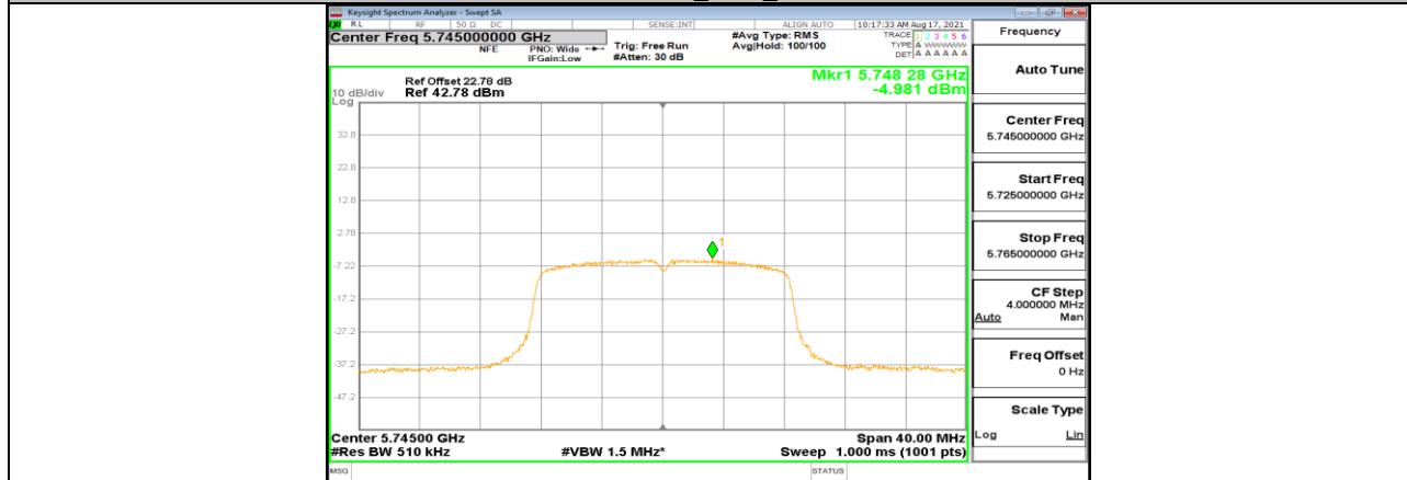
11A-CDD_Ant2_5745
