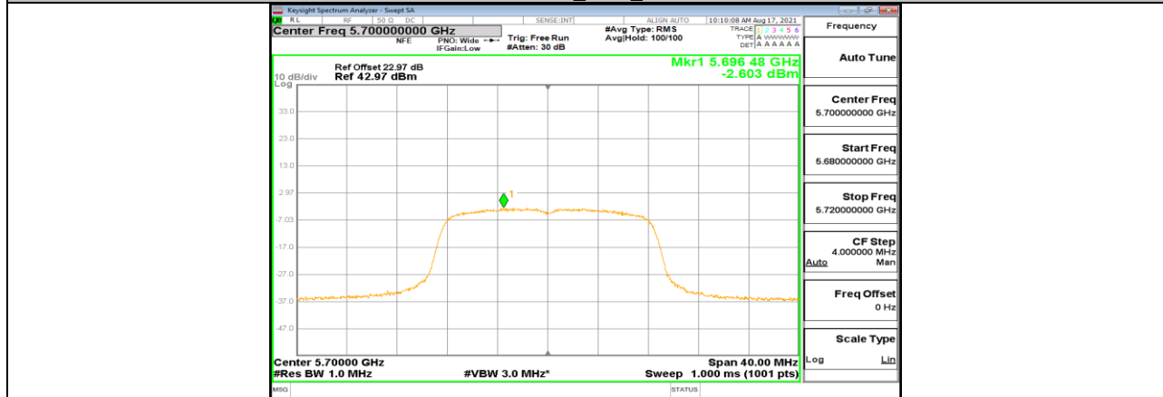
11A-CDD_Ant2_5700
