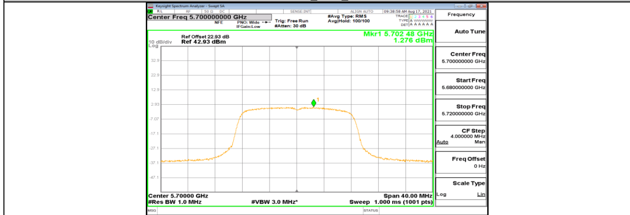
11A-CDD_Ant1_5700
