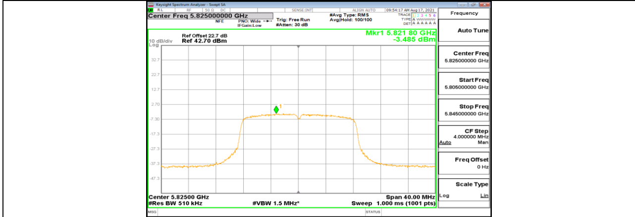
11A-CDD_Ant1_5825
