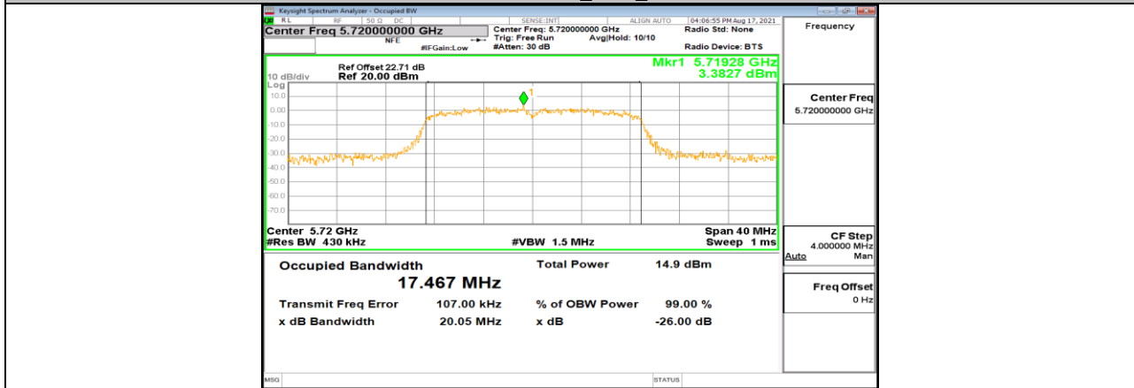
11AC20MIMO_Ant2_5720
