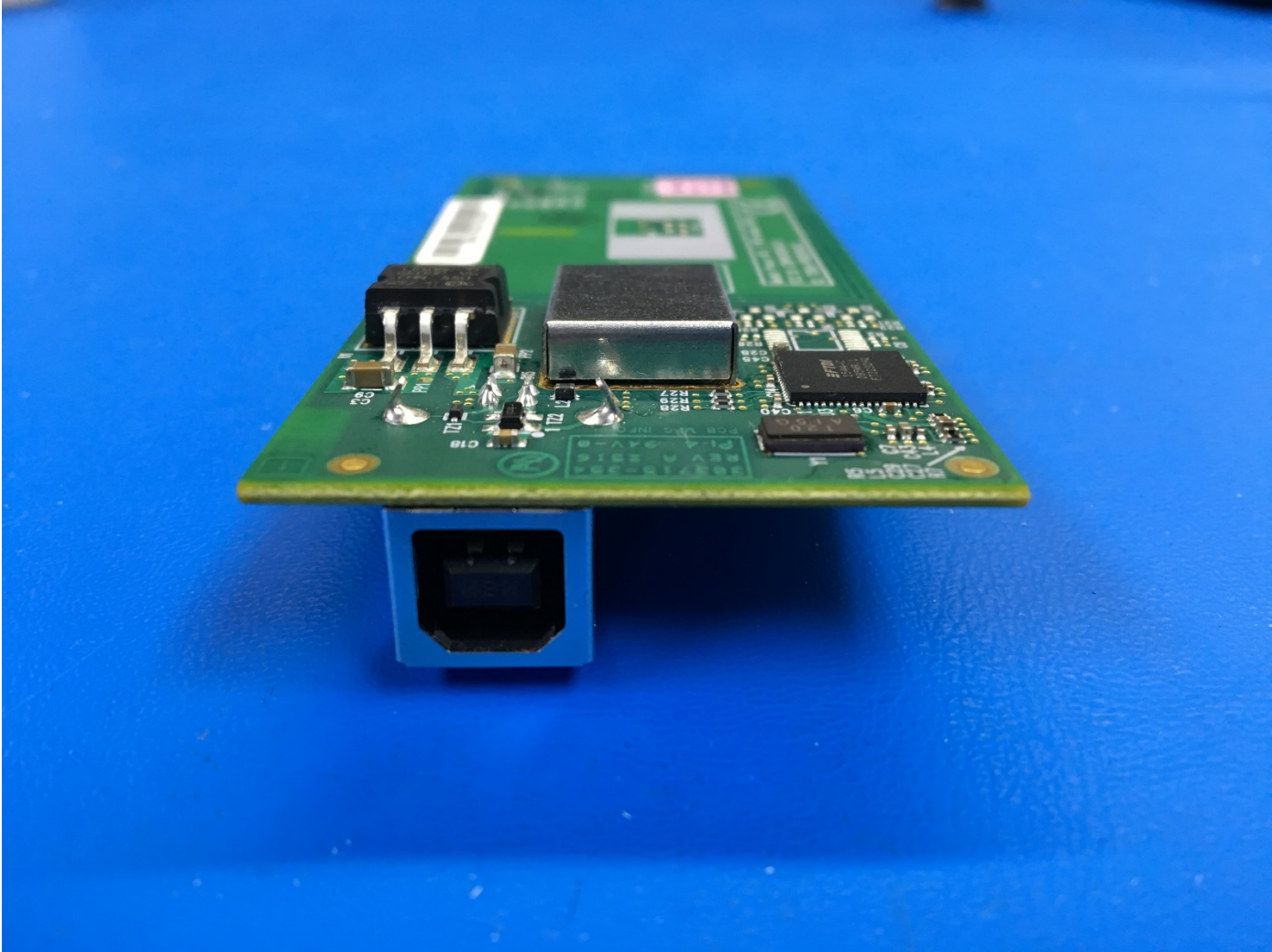
Precor NFC / RFID Module 304232 internal photos
