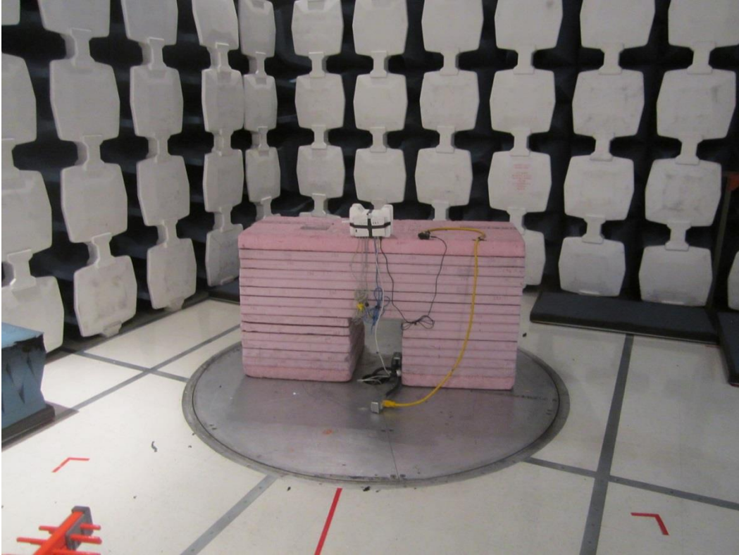
30MHz – 1GHz (EUT in Y orientation – EUT antenna horizontal)
