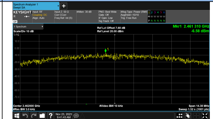
IEEE 802.11b - 2462MHz
