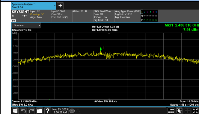
IEEE 802.11b - 2437MHz
