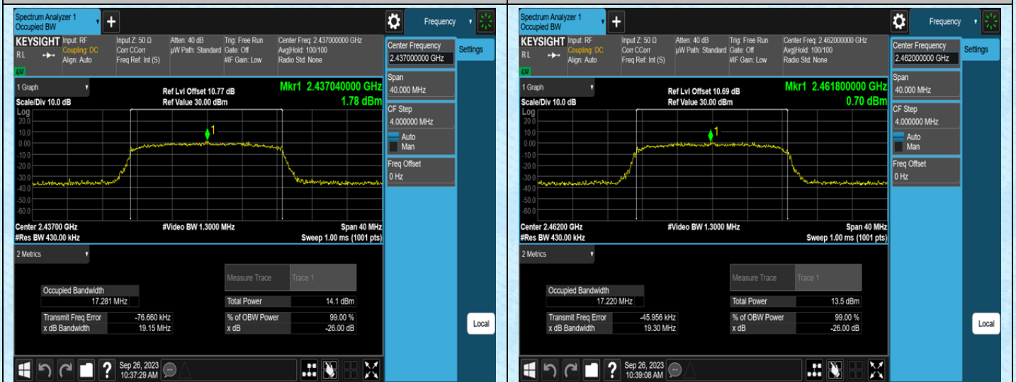
11G-Ant1-2437
