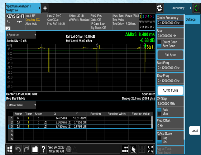
NTNV-P10-Ant1-2412
