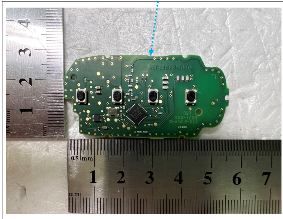
Antenna
