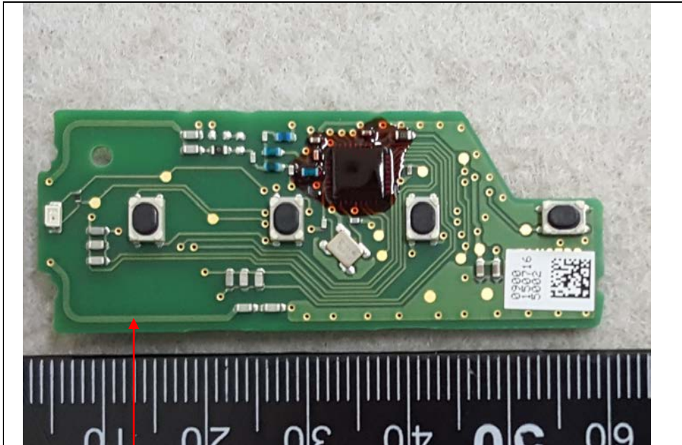
Antenna
