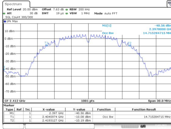
OBW NVNT b 2412MHz Ant1
