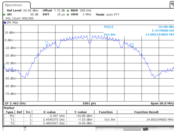
OBW NVNT b 2462MHz Ant1
