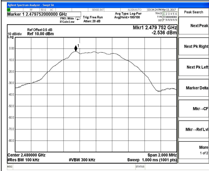
2479 – 2481 MHz
