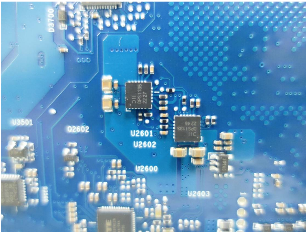
(46) EUT Photo
