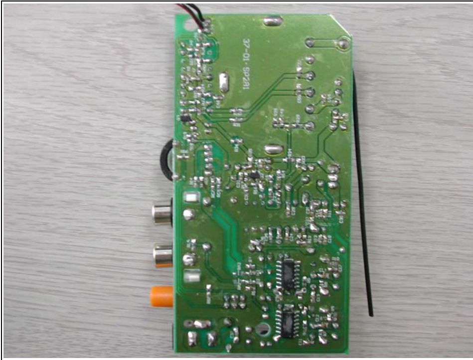
EUT Photo
