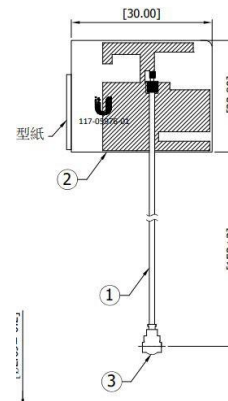
Antenna type: PIFA
