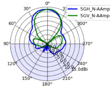
Elevation - 90.0°
