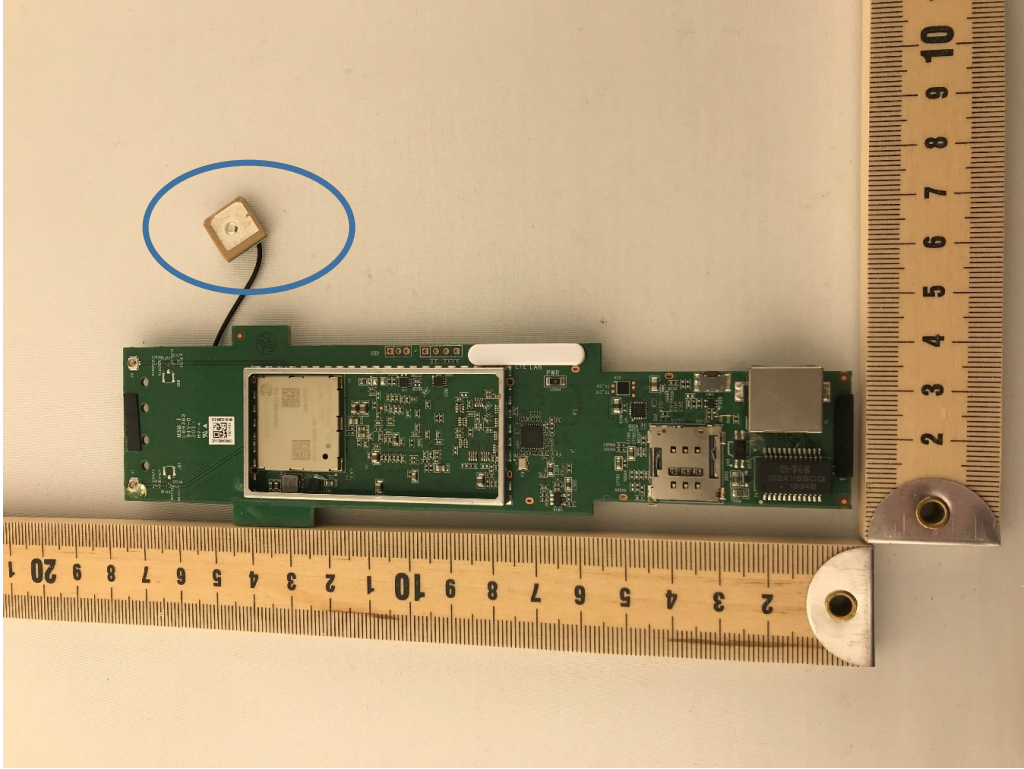
GPS Antenna
