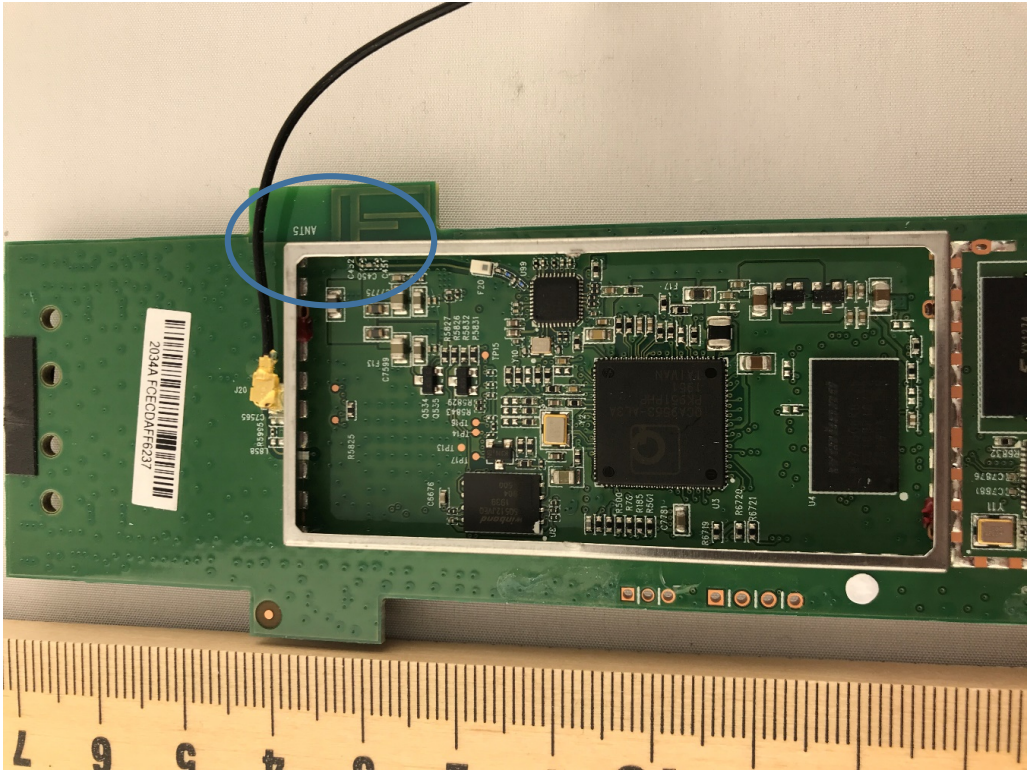
BLE Antenna
