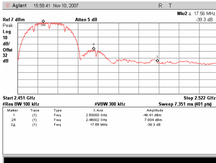
Plot 42. 802.11/b –Upper Band Edge
