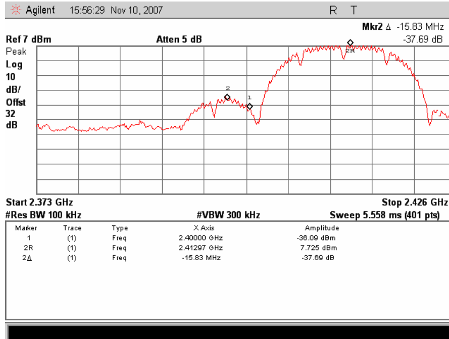
Plot 41. 802.11/b – Lower Band Edge
