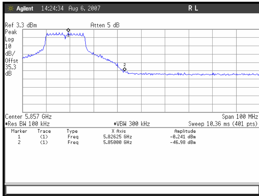
Plot 46. 802.11/a – Upper Band Edge
