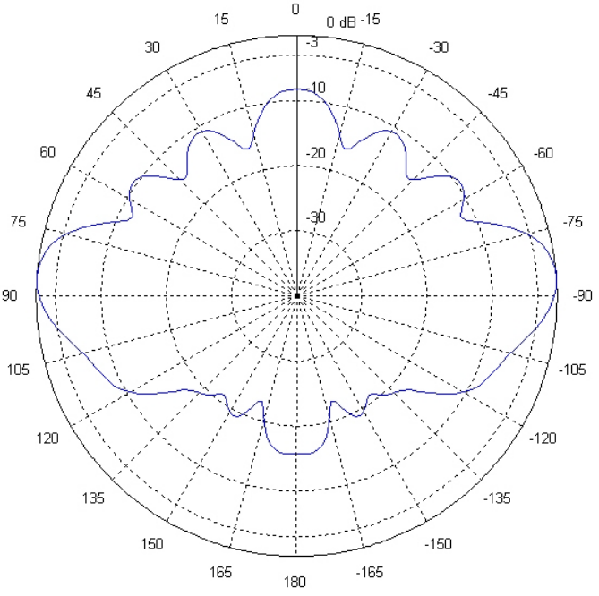
PAWMA9-7 7dBi E-Plane
