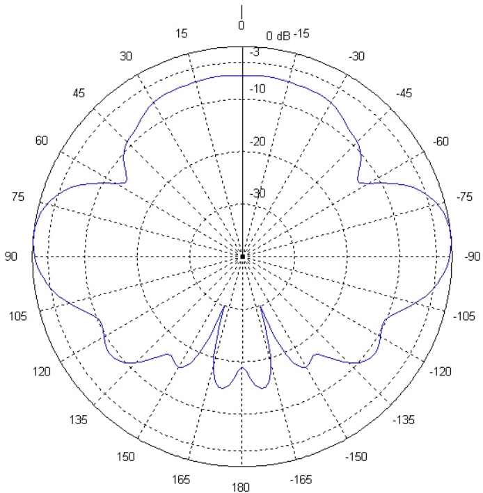
PAWMA9-5 5.5dBi E-Plane
