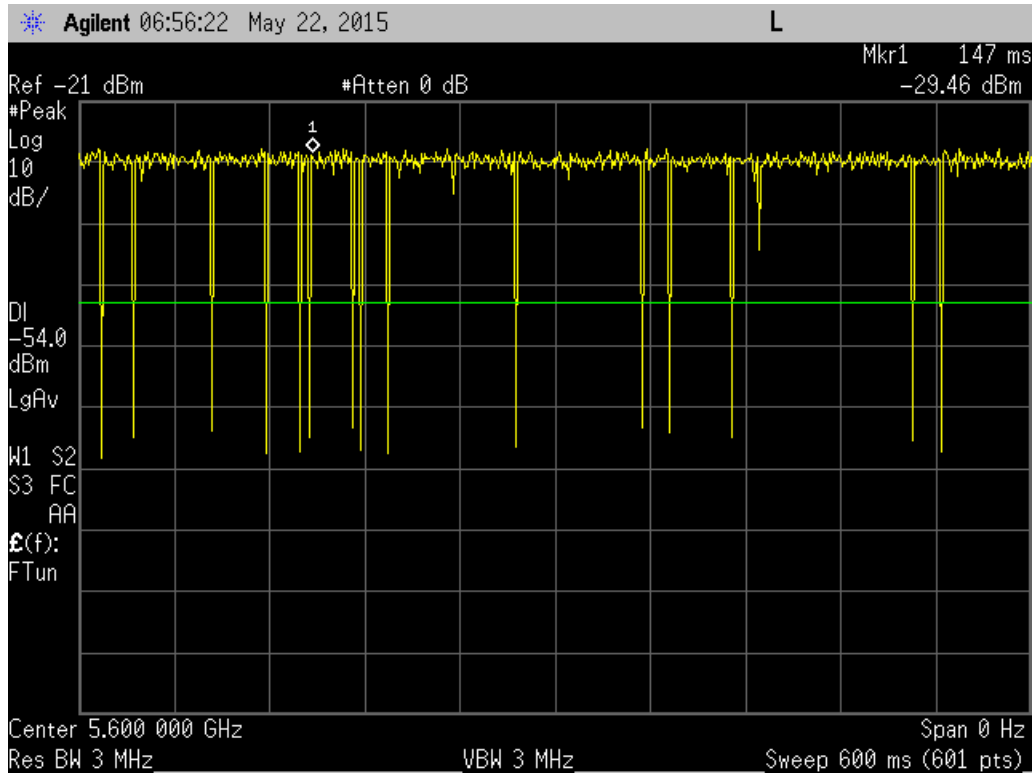
20MHz BW
