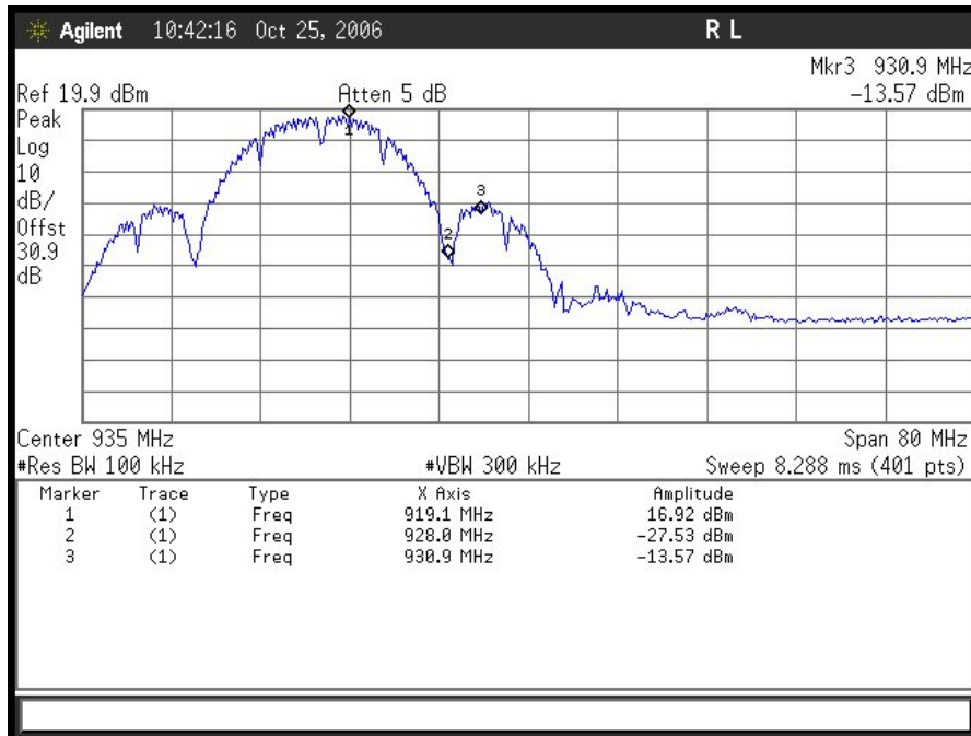
Plot 26. 802.11/g – 917MHz Upper Band Edge (DSSS 20MHz)
