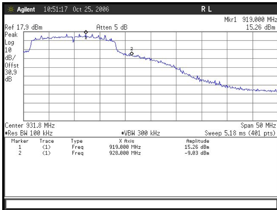
Plot 22. 802.11/b – 917MHz Upper Band Edge (OFDM 20MHz)
