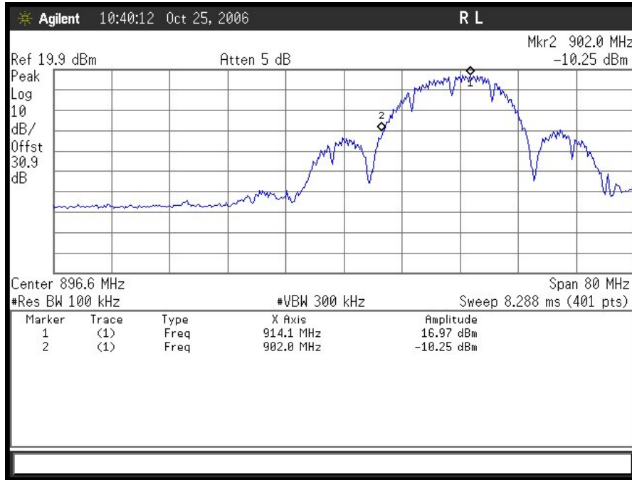
Plot 25. 802.11/g – 912MHz Lower Band Edge (DSSS 20MHz)
