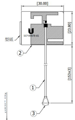
Antenna type: PIFA
