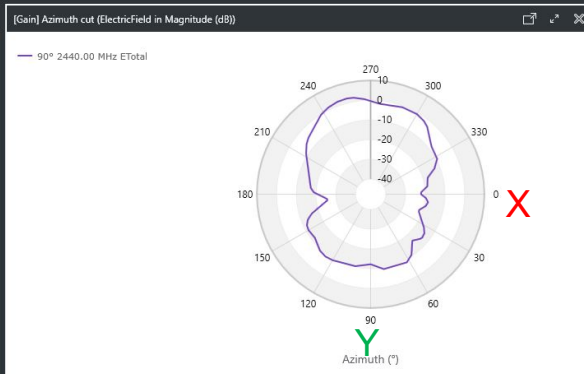
Antenna type: PIFA
