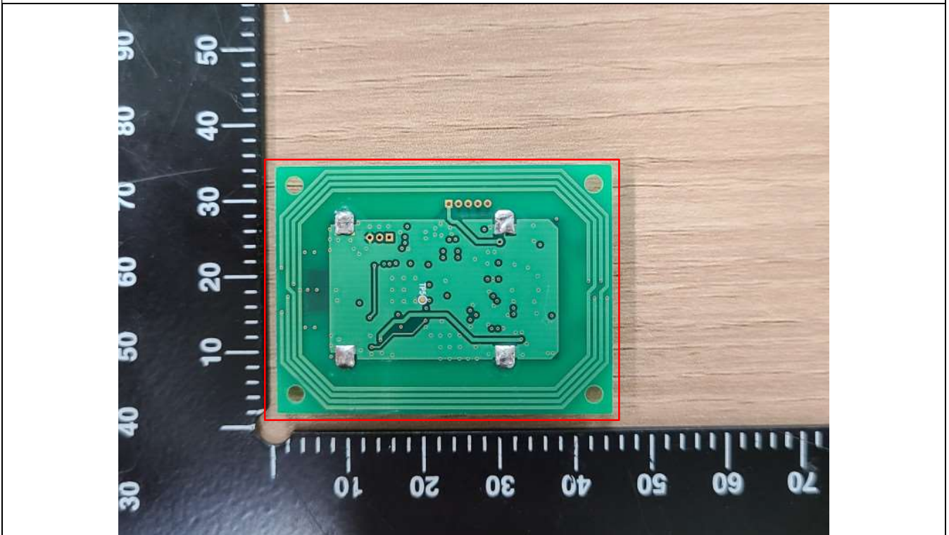
RFID Antenna
