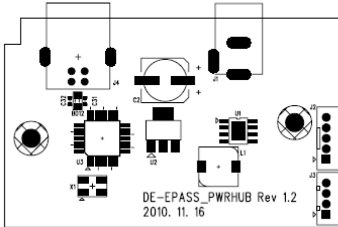
DE-EPASS_PWRHUB 보드 TOP side 부품배치도
