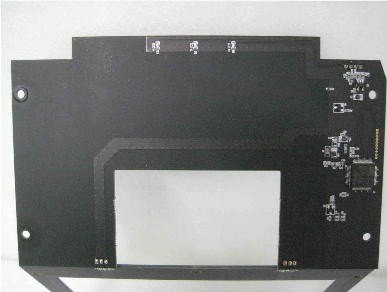
메인 보드 후면
